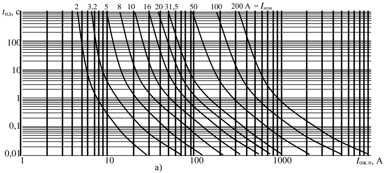
Рис. 5.5. Время-токовые характеристики плавких предохранителей группы
