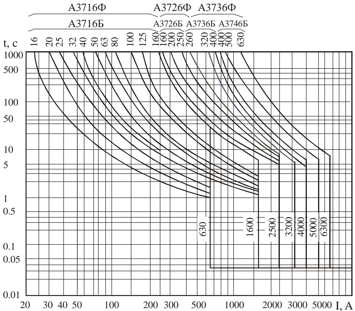
Рис. 4.8. Семейство защитных характеристик автоматических выключателей А3700 с комбинированными (термобиметаллическими и электромагнитными) расцепителями в исполнении токоограничивающем – А3700Б и нетокоограничивающем – А3700Ф.
